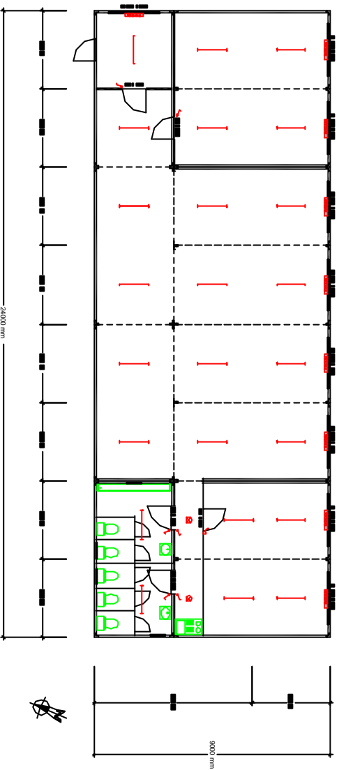
GRUNDRISSZEICHNUNG:
