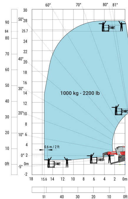
Drehung an abgesenkten Stützen mit 1000 kg Arbeitskorb
